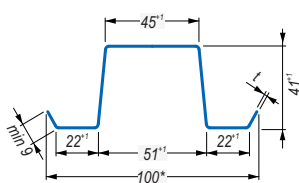
Обрешеточный профиль (ОП)
